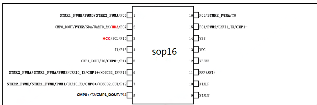
图 1-1 TX8W7011S016C 引脚图
