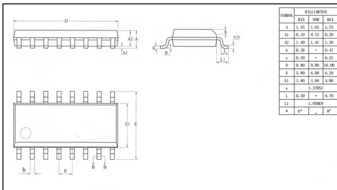
图 1-2 SOP16 封装 POD 图
