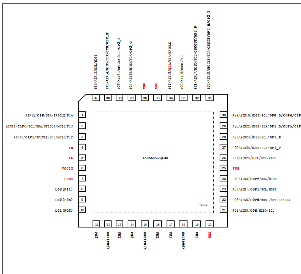
图 2 - TX8M2262QF40 (QFN40) 封装图
