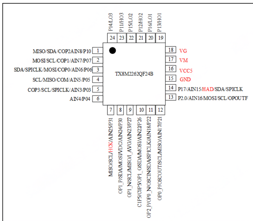
图 1 - TX8M2262QF24B (QFN24) 封装图
