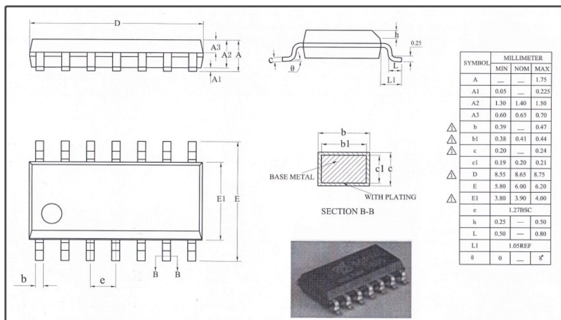
图 1-6 SOP14 封装 POD 图
