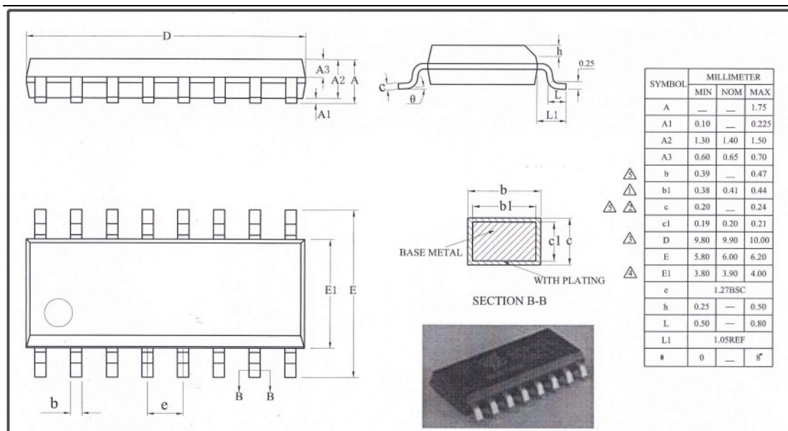
图 1-7 SOP16 封装 POD 图
