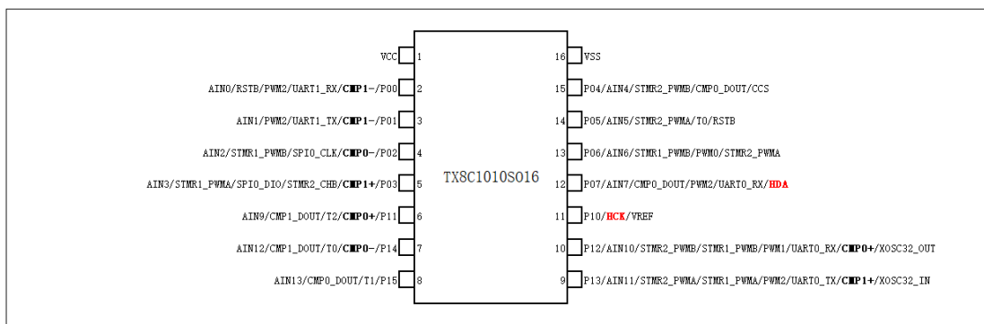
图 1-3 TX8C1010S016（SOP16）引脚图
