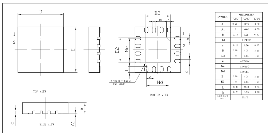
图 1-8 QFN16 封装 POD 图
