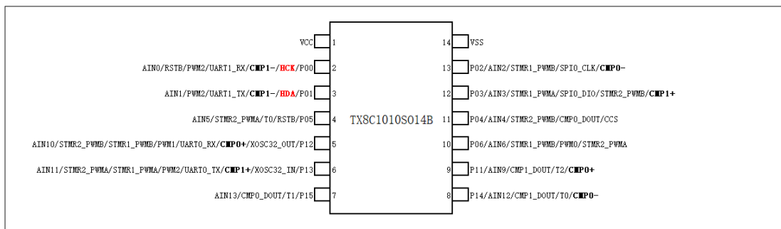
图 1-2 TX8C1010S014B（SOP14）引脚图
