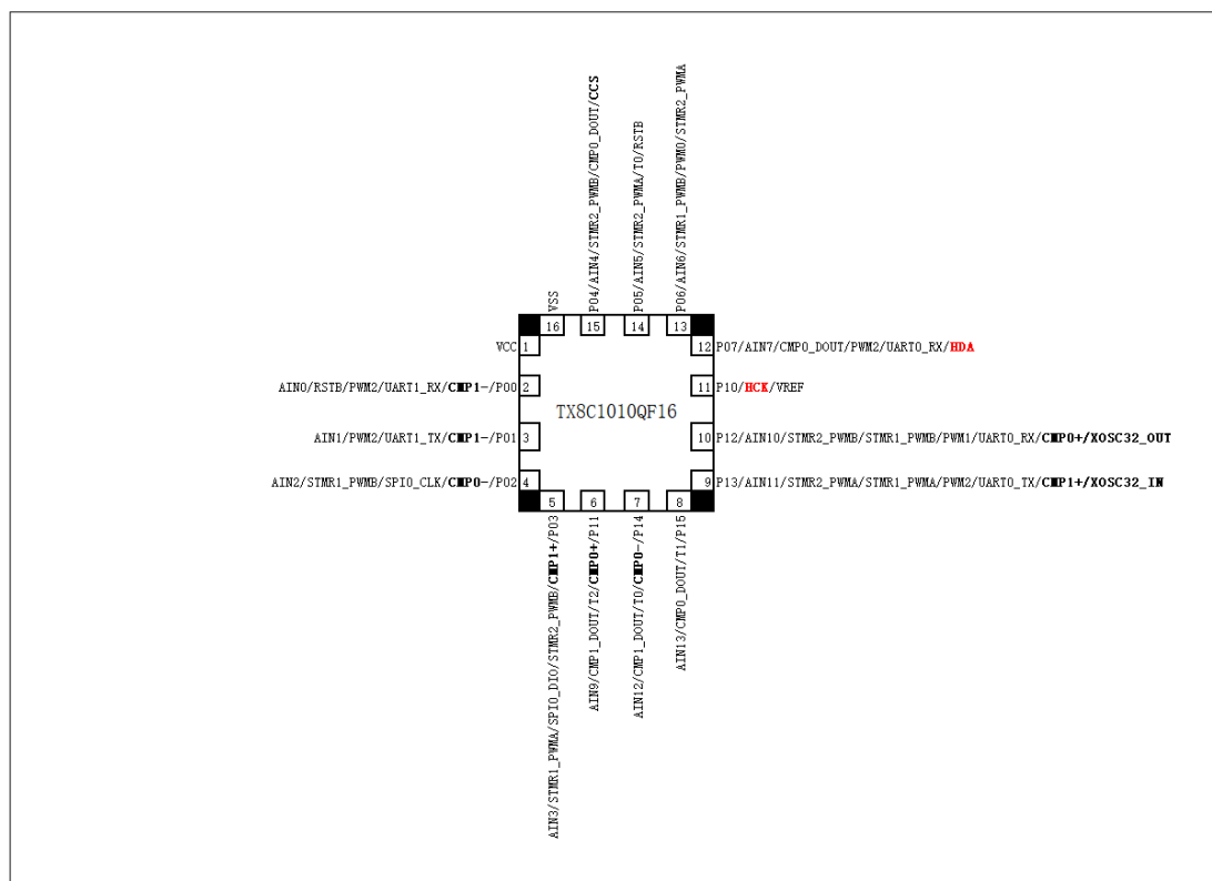
图 1-4 TX8C1010QF16 引脚图
