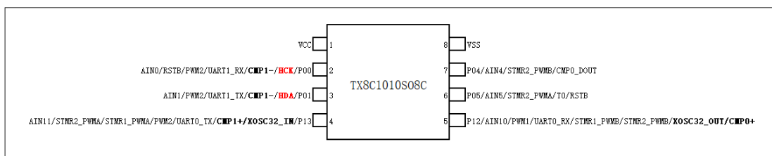
图 1-1 TX8C1010S008C（SOP8）引脚图
