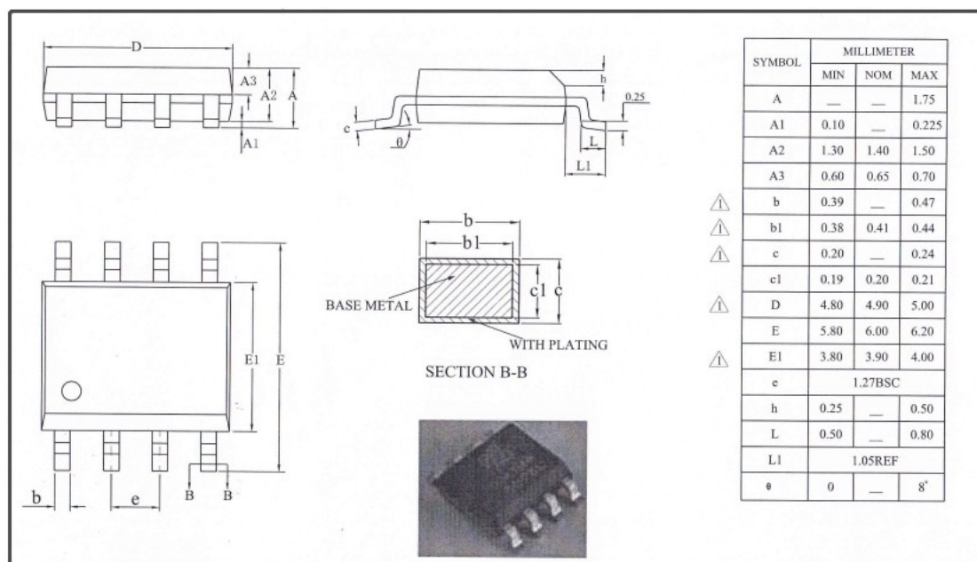
图 1-5 SOP8 封装 POD 图
